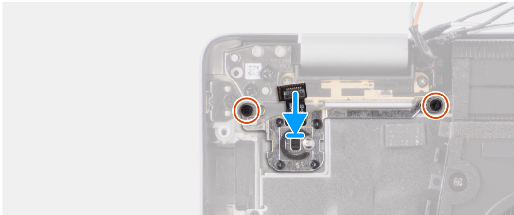
Abbildung 74. Installieren des Netzschalters mit optionalem Fingerabdruck-Lesegerät
