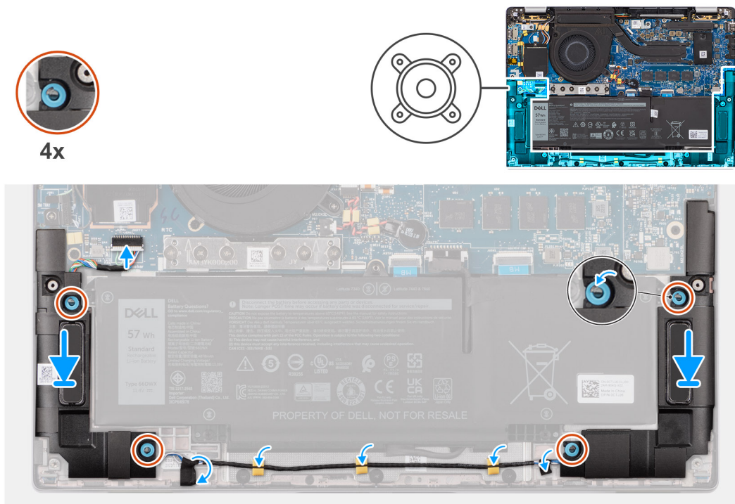
Abbildung 31. Installieren der Lautsprecher (Mainstream)
