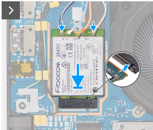
Abbildung 22. Installieren der 4G-WWAN-Karte
