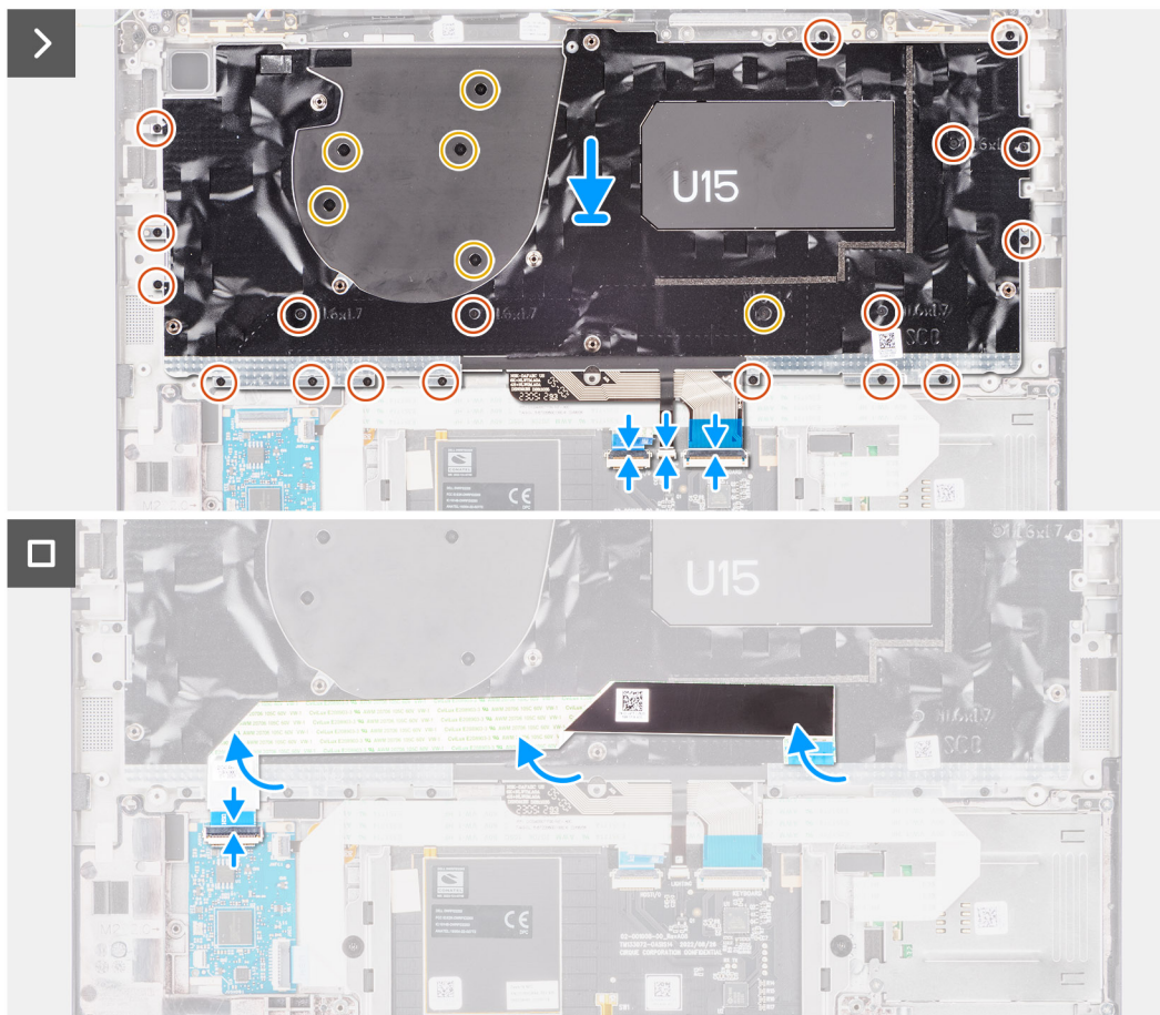
Abbildung 78. Installieren der Tastatur
