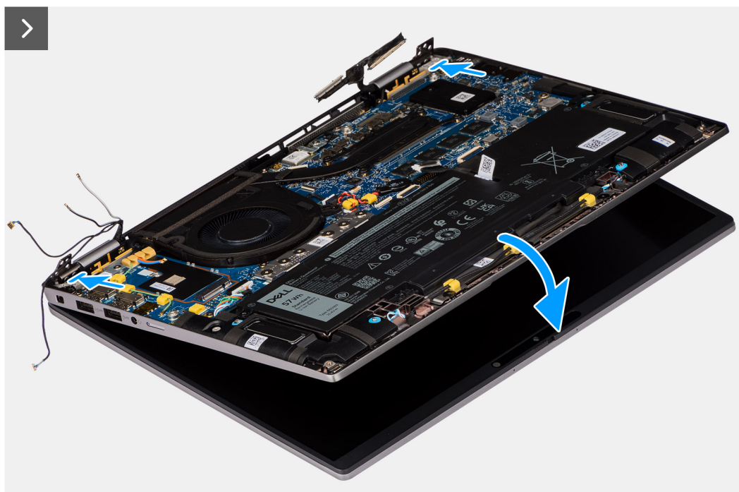
Abbildung 50. Installieren der Displaybaugruppe
