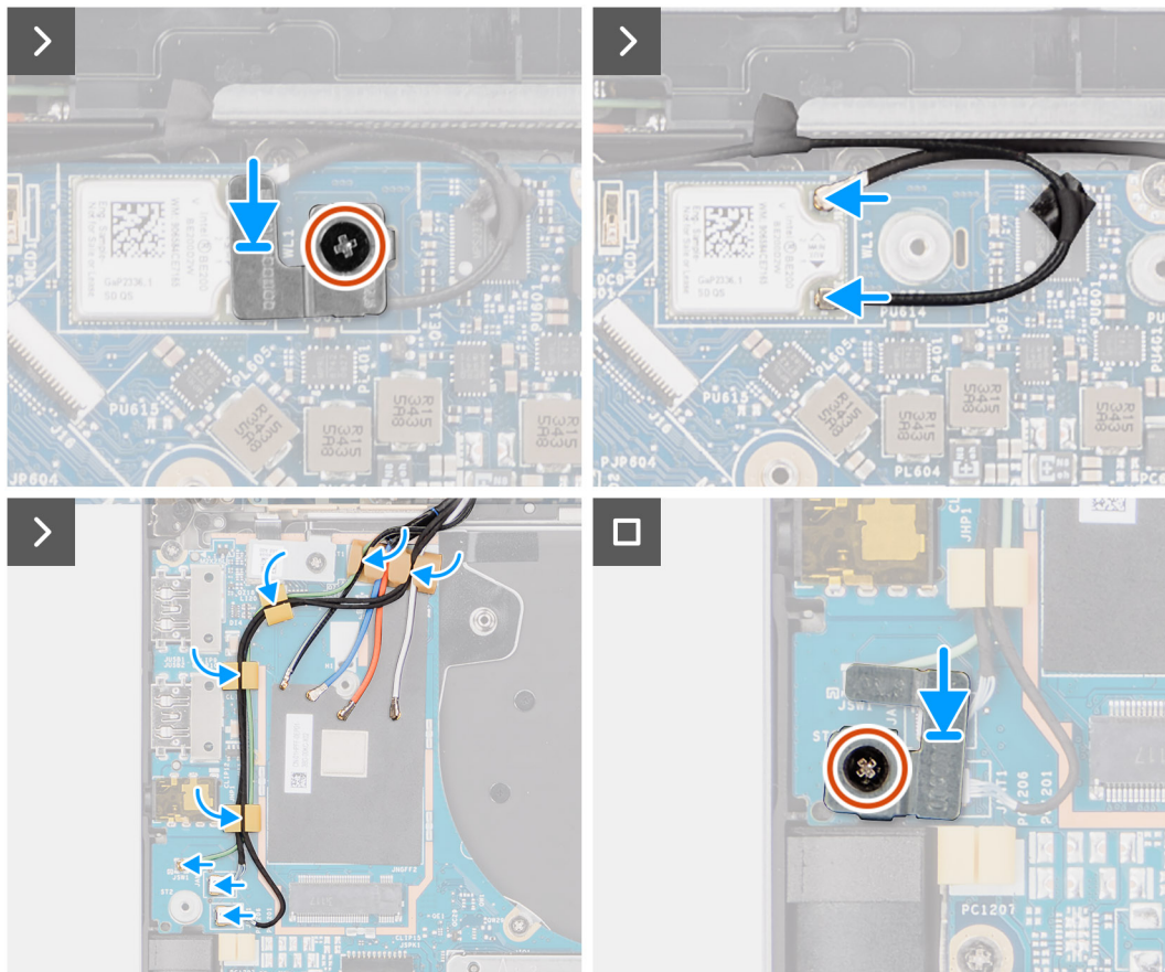
Abbildung 66. Installieren des WLAN-Antennenmoduls
