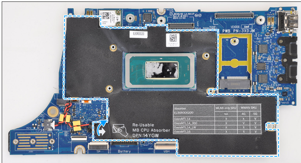
Abbildung 58. CPU-Absorber
